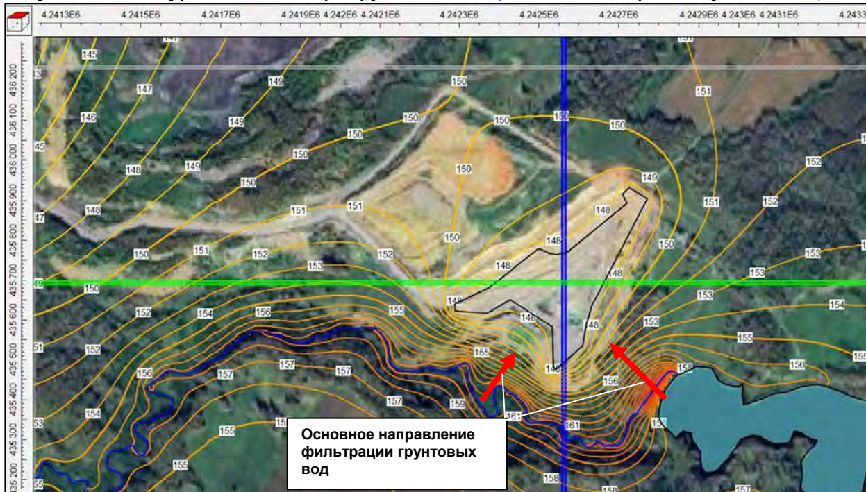
Рисунок 6 – Контурное поле напора грунтовых вод. Карьер «Выдрихинский»
