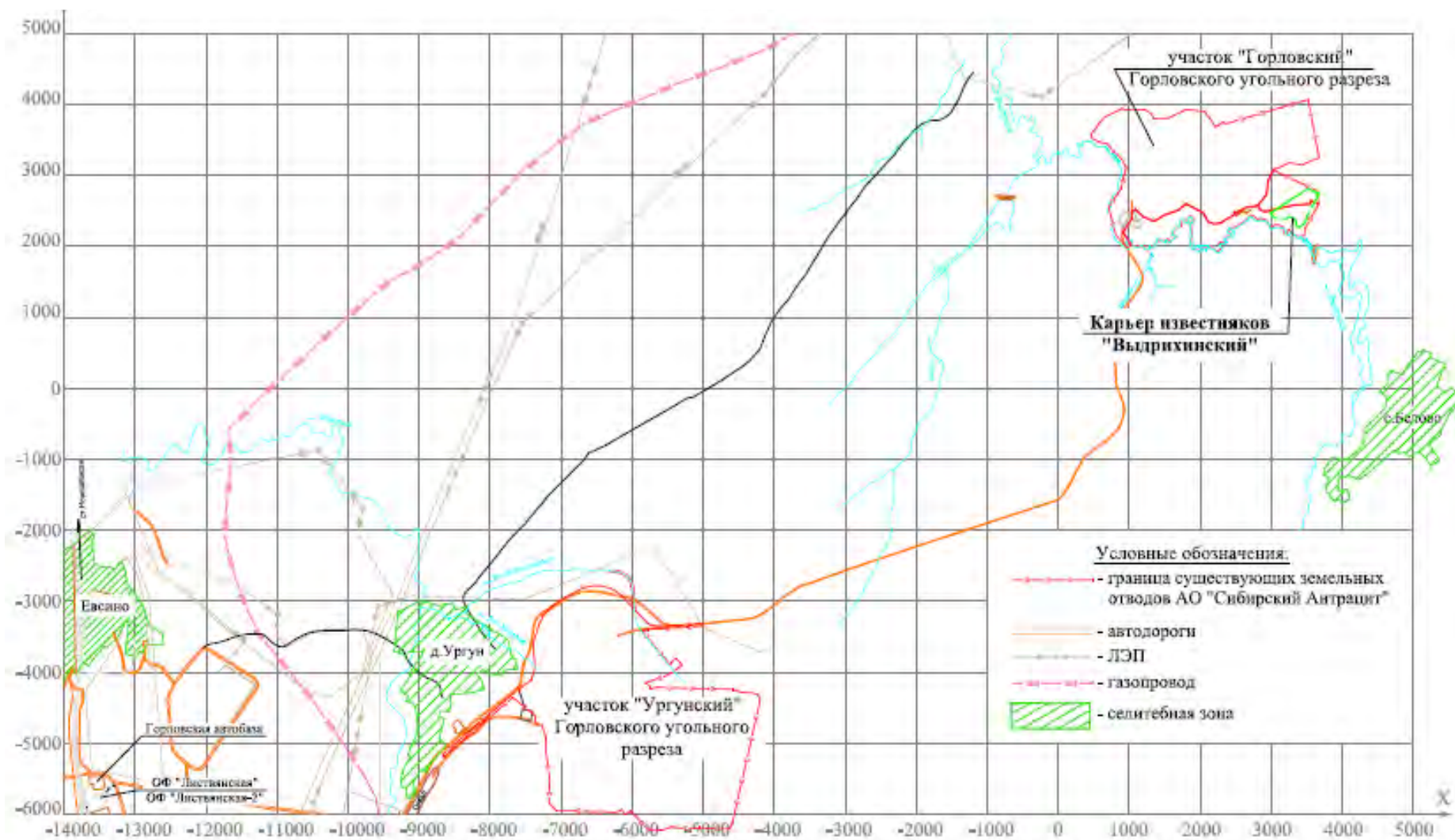
Рисунок 2.1 - Ситуационная схема расположения объекта
