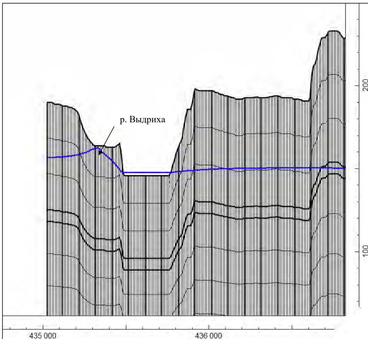
Рисунок 8 – Уровень грунтовых вод карьера «Выдрихинский». Разрез по синей линии (см. рисунок 6) (масштаб по оси Z увеличен в 10 раз)
