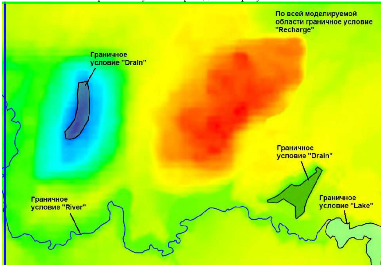
Рисунок 4 – Граничные условия математической модели
