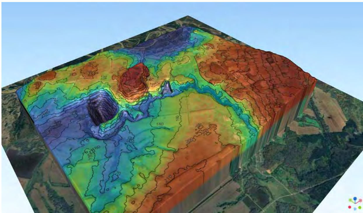
Рисунок 1 – Цифровая модель рельефа (3D-вид. Координаты Z увеличены в 5 раз)
